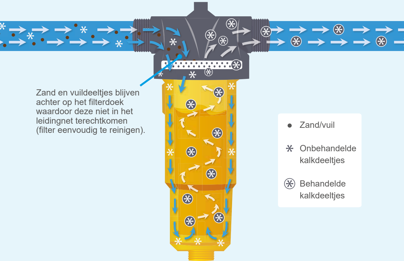
Doseringsunit met geïntegreerd filterdoek
